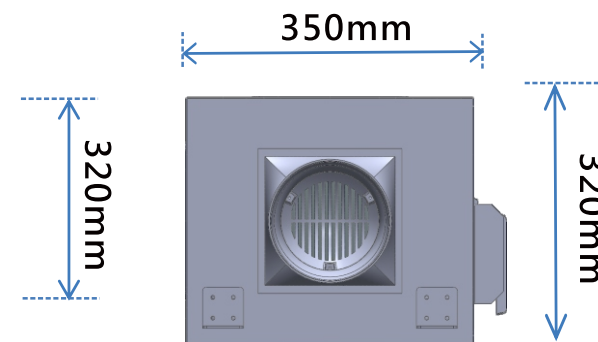
正視圖
