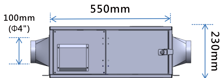
側視圖
