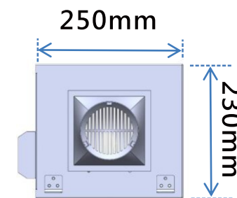
正視圖
